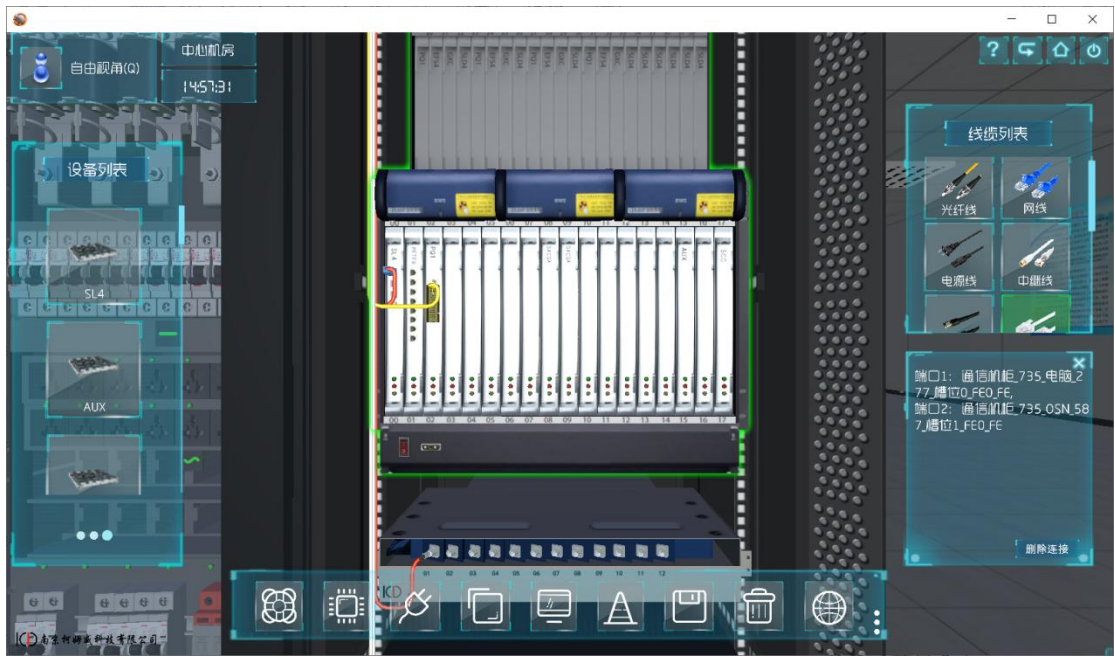
图 3.7 设备连线
